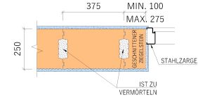
- VERBUND AN DER TÜRLAIBUNG, 2. REIHE DES MAUERWERKS
